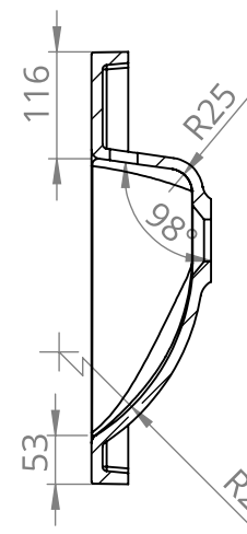
PRZEKRÓJ M-M SKALA 1 : 9
