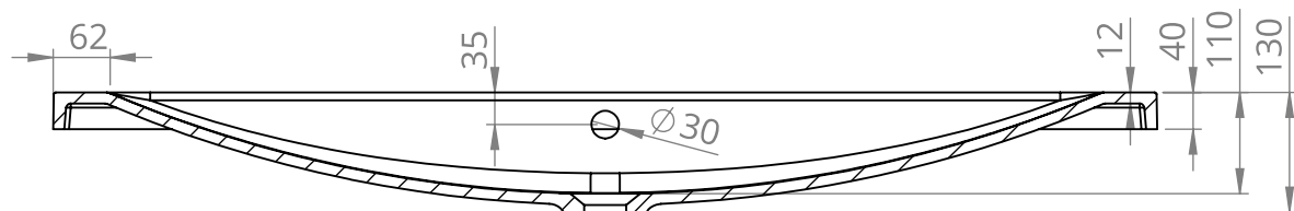
PRZEKRÓJ M-M SKALA 1 : 9
